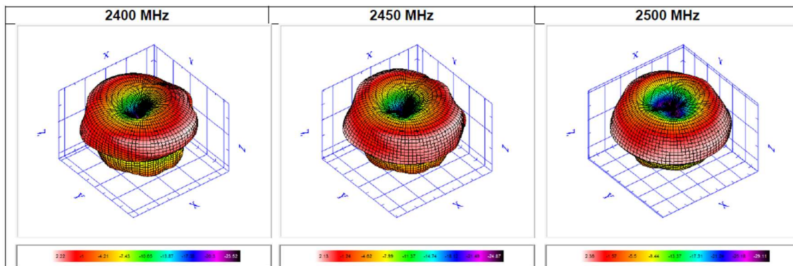
YAGEO : ANTX100ETHAB24553
